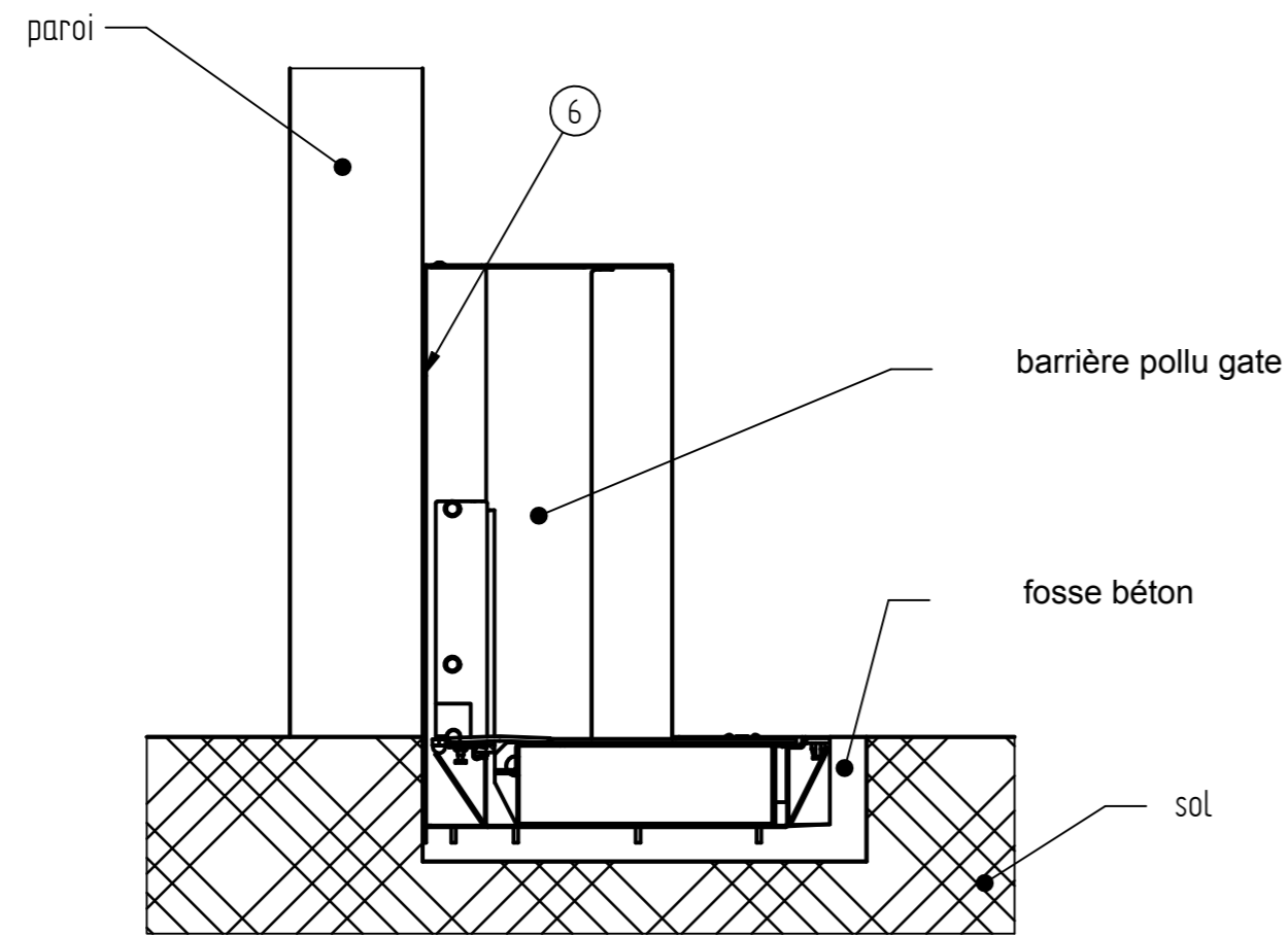
Schnitt B-B
