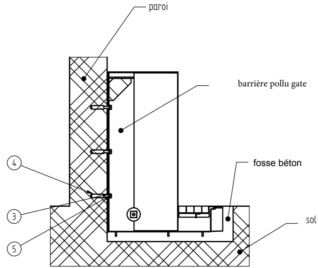
Schnitt C-C
