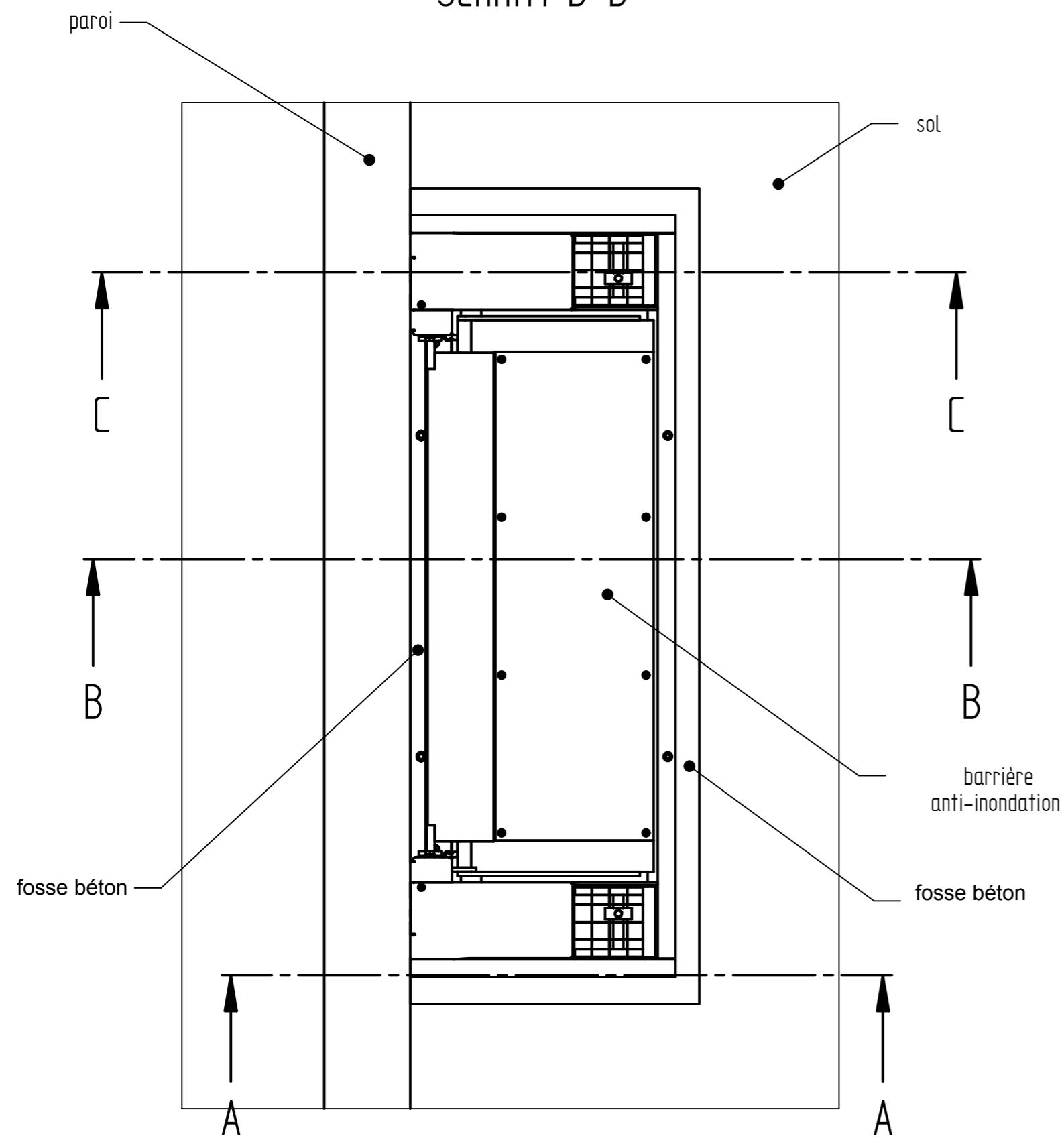
Schnitt B-B
